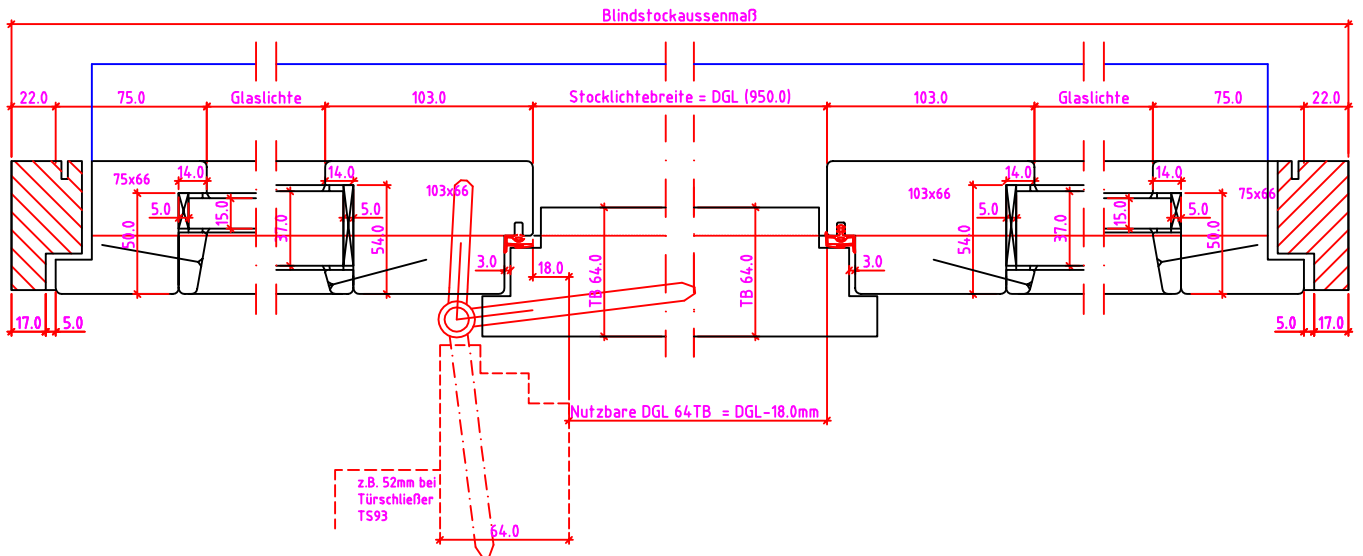
32mm Niveauunterschied
