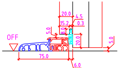
ohne Niveauunterschied
