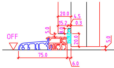
ohne Niveauunterschied
