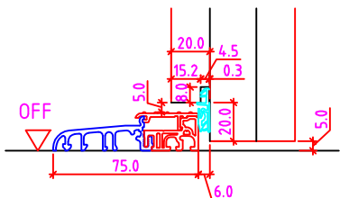
ohne Niveauunterschied
