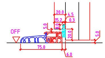
ohne Niveauunterschied
