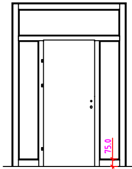
RST 2SK Anschlag links
