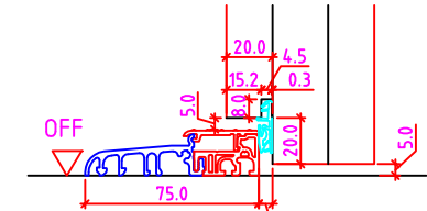
ohne Niveauunterschied
