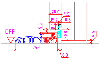
ohne Niveauunterschied
