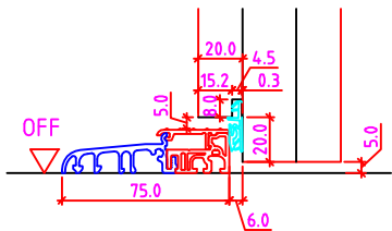
ohne Niveauunterschied
