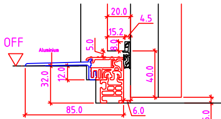
32mm Niveauunterschied
