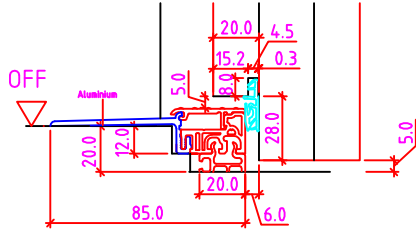
20mm Niveauunterschied
