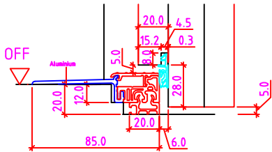
20mm Niveauunterschied
