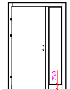
RST 1S-R Anschlag links
