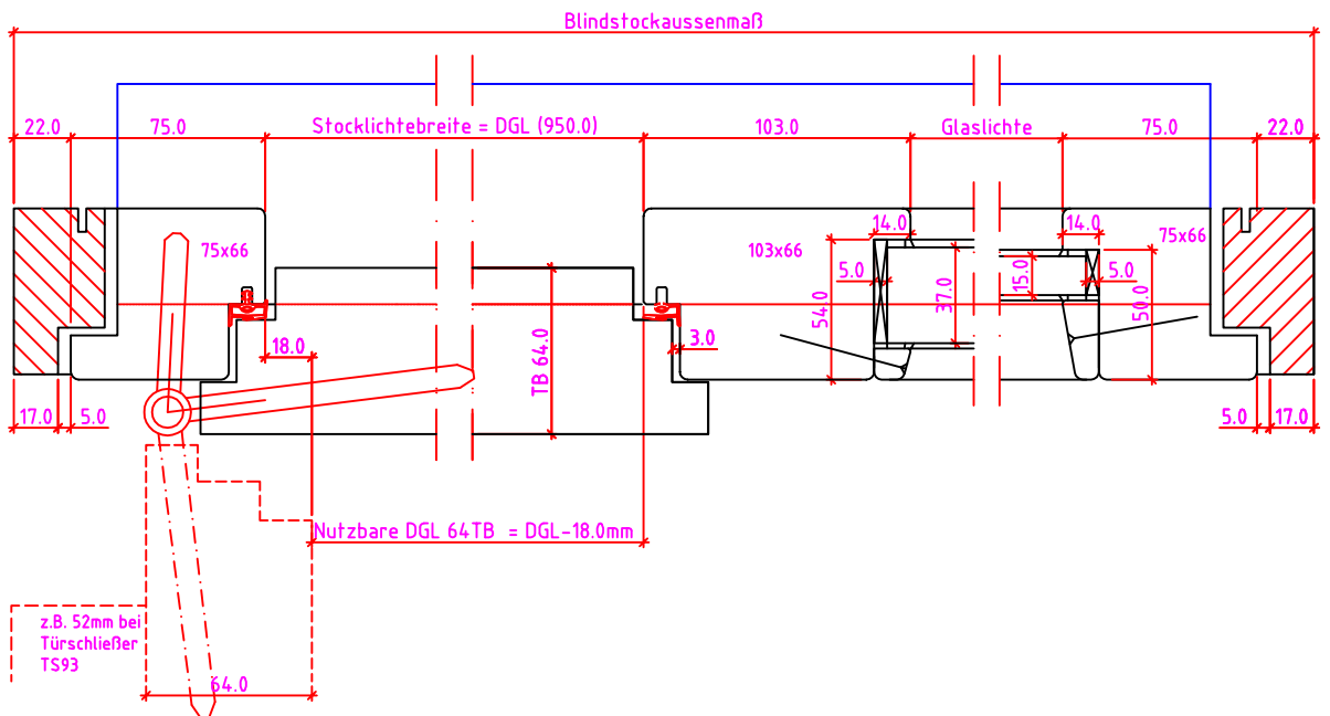
32mm Niveauunterschied
