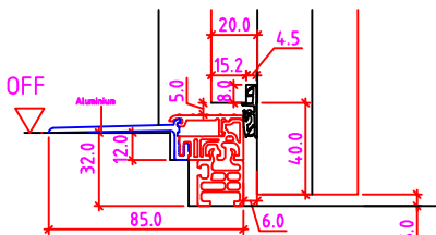
32mm Niveauunterschied
