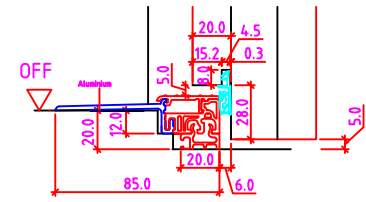
20mm Niveauunterschied
