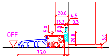
ohne Niveauunterschied
