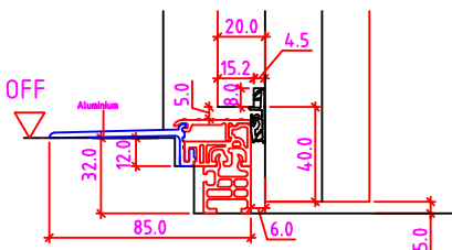
32mm Niveauunterschied
