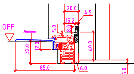
32mm Niveauunterschied
