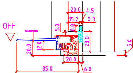
20mm Niveauunterschied
