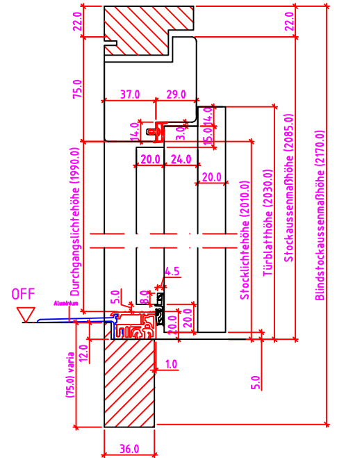
12mm Niveauunterschied
