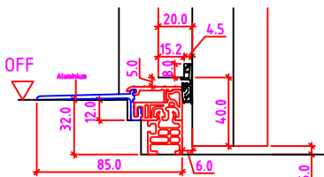
32mm Niveauunterschied
