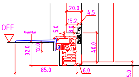
32mm Niveauunterschied
