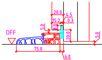
ohne Niveauunterschied
