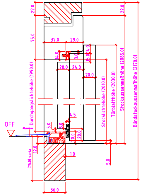
12mm Niveauunterschied
