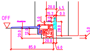
20mm Niveauunterschied
