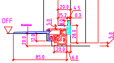
20mm Niveauunterschied
