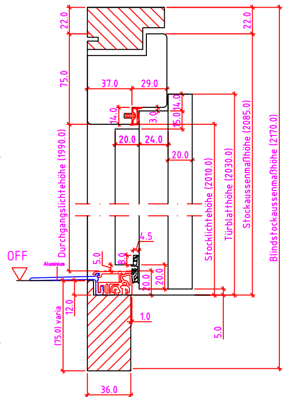
12mm Niveauunterschied
