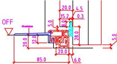
20mm Niveauunterschied
