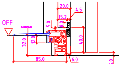
32mm Niveauunterschied
