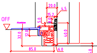
32mm Niveauunterschied
