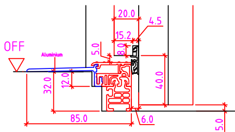
32mm Niveauunterschied
