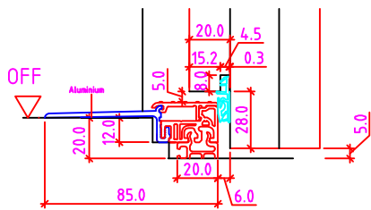
20mm Niveauunterschied
