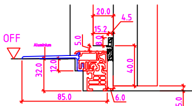
32mm Niveauunterschied
