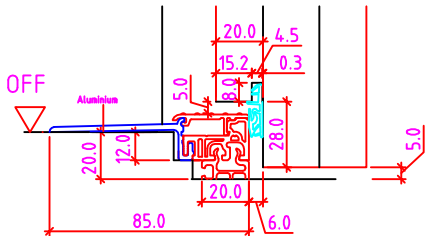
20mm Niveauunterschied
