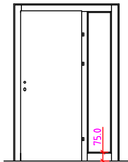
RST 1S-R Anschlag rechts
