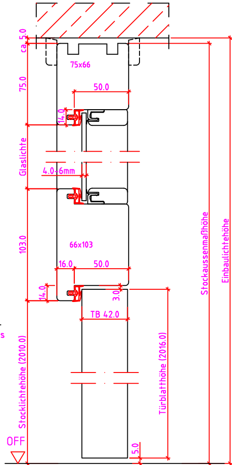
RST 1SK-R Anschlag rechts
