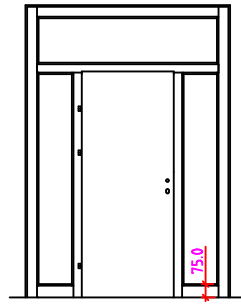
RST 2SK Anschlag links
