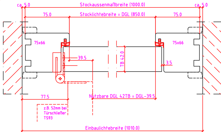
40.0 Bodeneinstand
