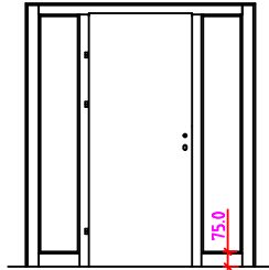
RST 2S Anschlag links
